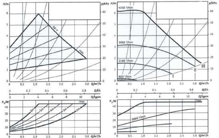
dp-v (variable Differenzdruckregelung)
