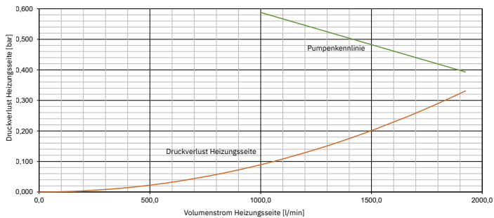
Volumenstrom der Primärseite bei verschiedenen Vorlauftemperaturen für die Trinkwassererwärmung
