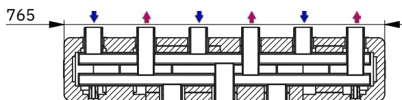
UNI 80/125-3 3 Heizgruppen
