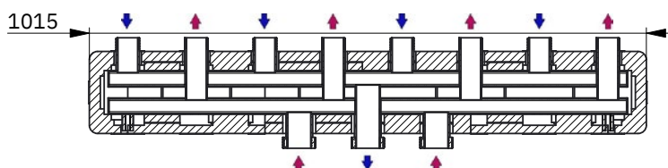
UNI 80/125-4 4 Heizgruppen
